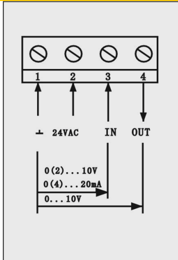
接线图
