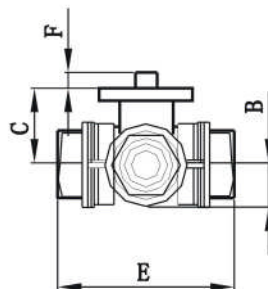
三通阀
