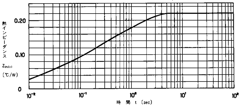
過渡熱インピーダンス (接合—ケース間、対総損失)
