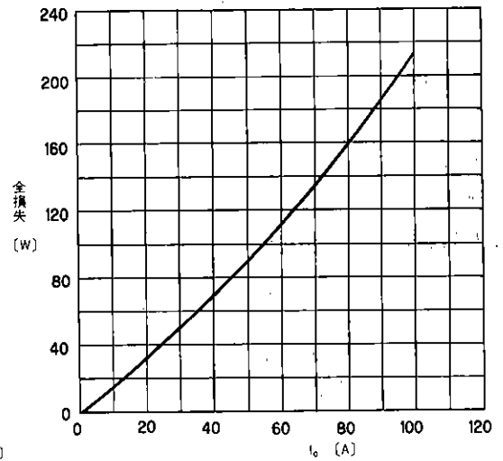
全損失 Total Loss
