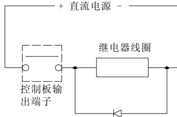
直流吸收电路
