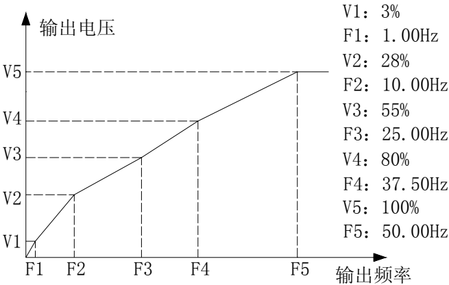
自设定V/F曲线示意图
