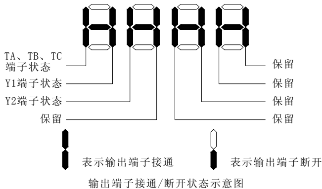
输出端子断开接通状态示意图
