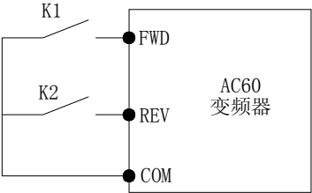
1. 二线式运转控制示意图
