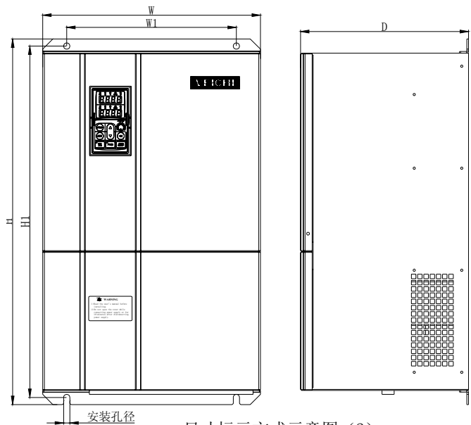
尺寸标示方式示意图（2）
