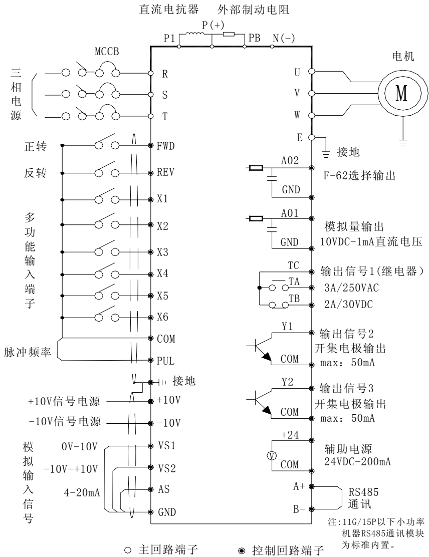
变频器基本配线示意图
