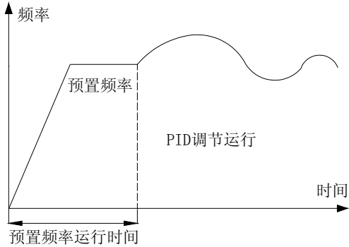
PID预置频率运行示意图
