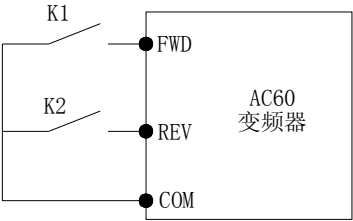
0. 标准运转控制示意图
