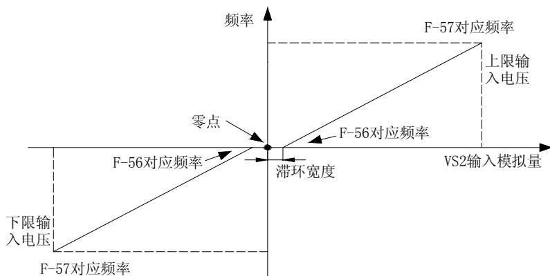
VS2双极性控制示意图
