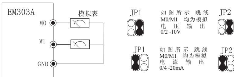
图 3-14 模拟输出端子配线
