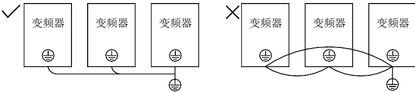
图 3-10 接地线连接方法
