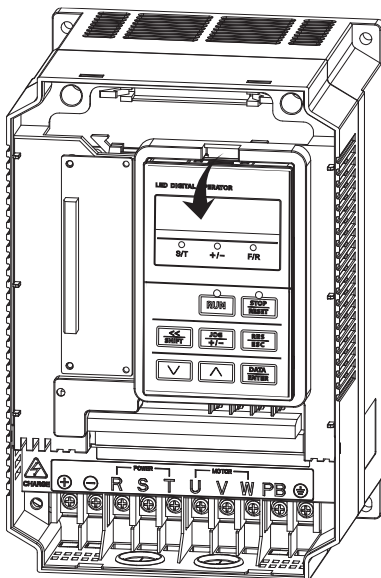
图 2-4 键盘拆卸图示
