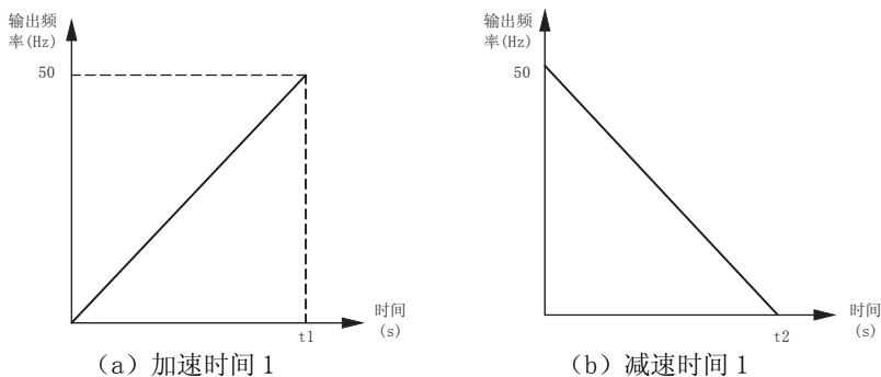
图 7-4 加减速时间
