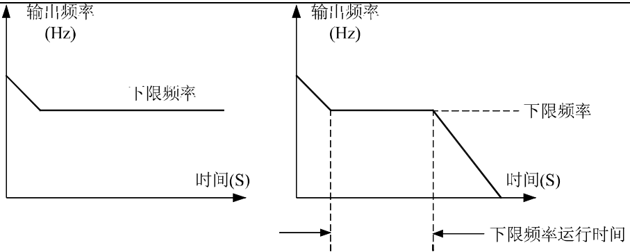
图 7-14 下限频率控制示意图
