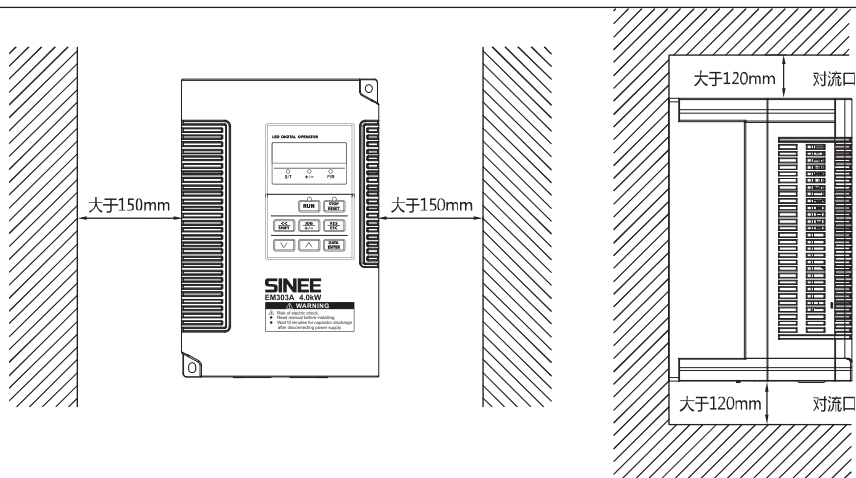
图 2-2 变频器安装方向和空间
