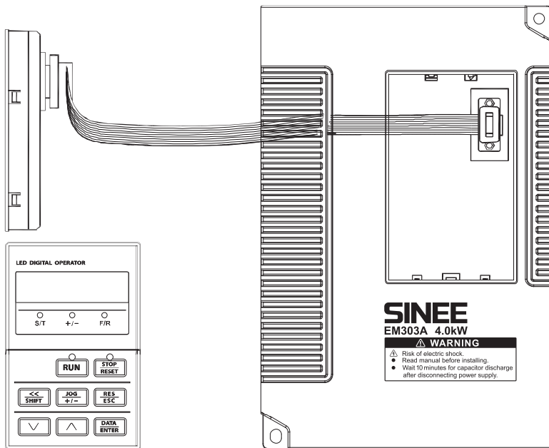
图 3-18 拉出键盘装延长线
