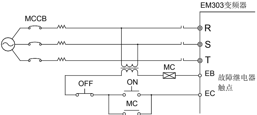
图 3-4 接入输入断路器
