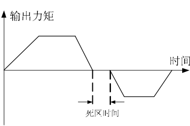
图 7-20 正/负力矩死区时间
