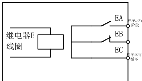
图 7-9 继电器触点
