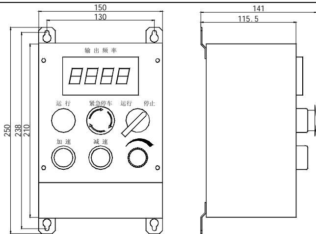
图 11-1 远程操作箱外形尺寸
