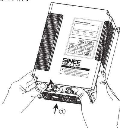
图 2-3 面板开启图示
