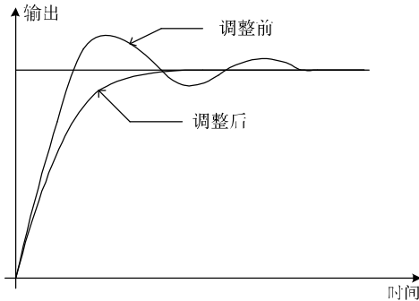
图 7-17 抑制输出超调
