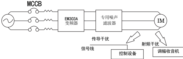
图 3-7 输出侧安装噪声滤波器
