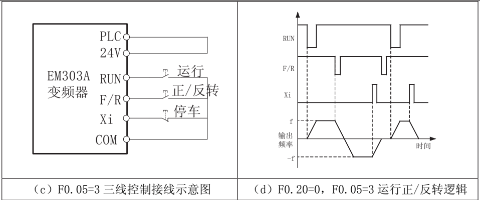
图 7-3 三线控制
