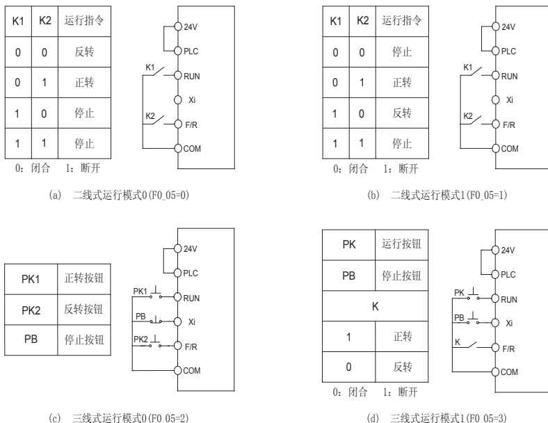
图 1-3 端子运行方式控制逻辑图
