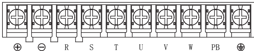
(a) 15kW 及以下规格主回路端子
