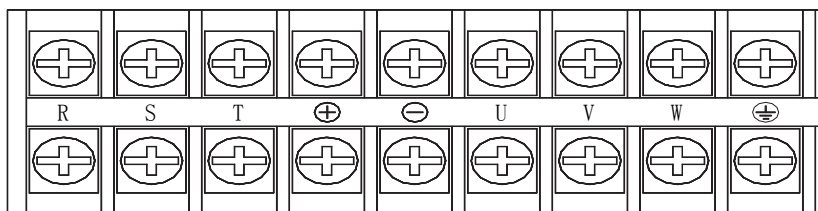
(b) 18.5~75kW 各规格主回路端子
