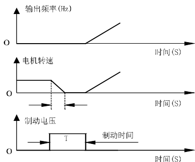
图 7-12 启动直流制动过程
