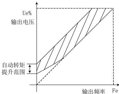
图 8-2 自动转矩提升
