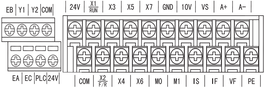
a. 控制回路端子
