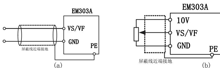
图 3-12 VS、VF 端子配线图
