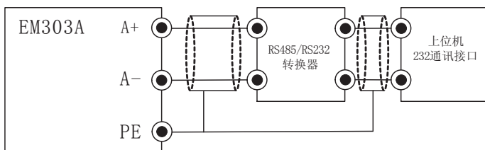
图 3-16 通讯端子配线
