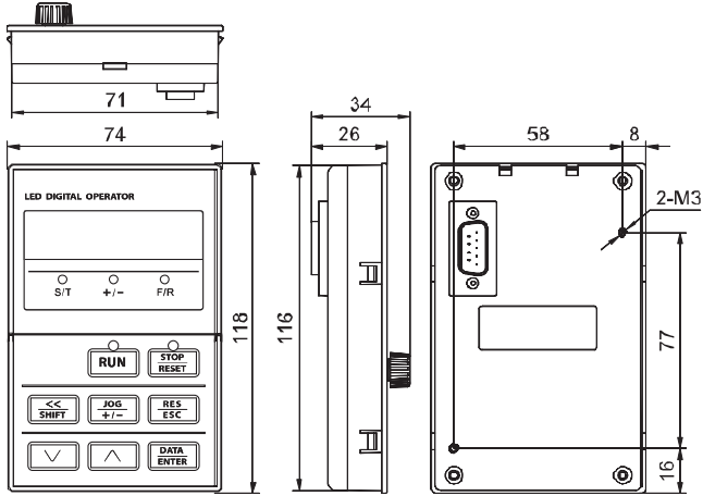
(a) 键盘尺寸
