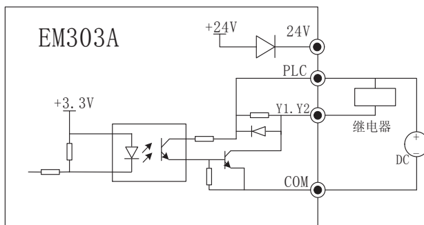
图 3-13 (b) 多功能输出端子用外部电源接线方式
