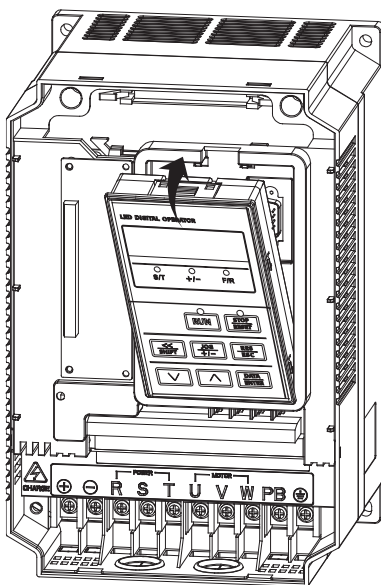
图 2-5 键盘安装图示
