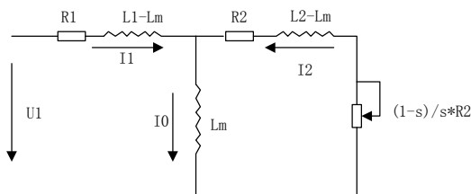
图 7-7 异步电动机稳态等效模型
