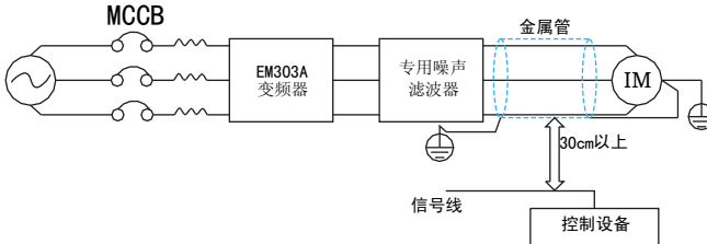
图 3-8 感应干扰对策
