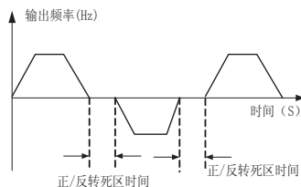
图 7-6 正/反转死区时间示意图
