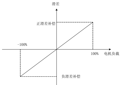
图 8-3 滑差补偿
