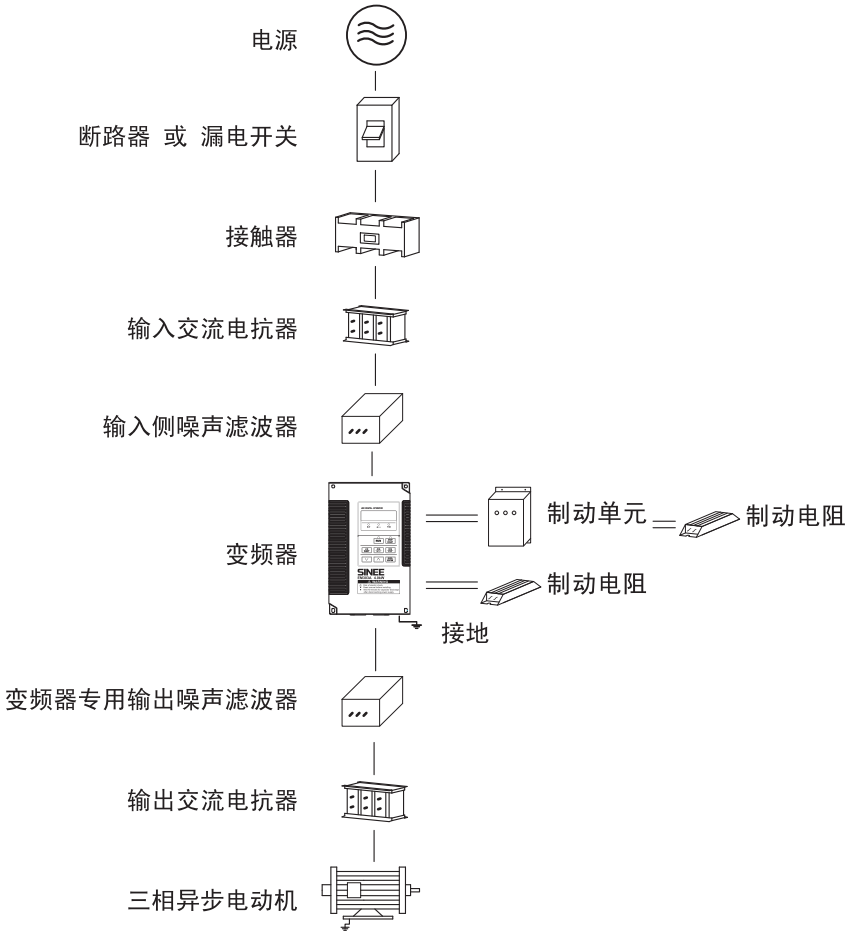
3-1 变频器与外围设备的连接图
