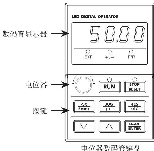
图 4-1 键盘各部件名称
