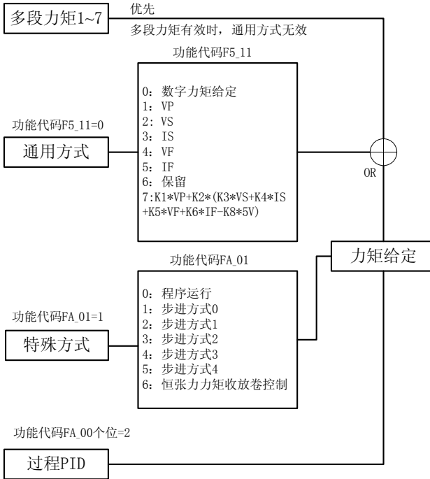
图 1-2 力矩输入方式示意图
