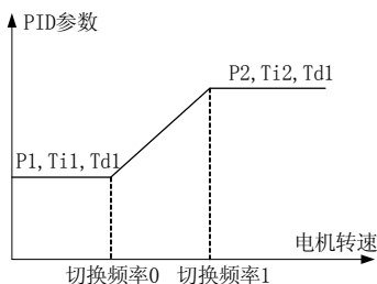
图 7-19 PID 参数示意图
