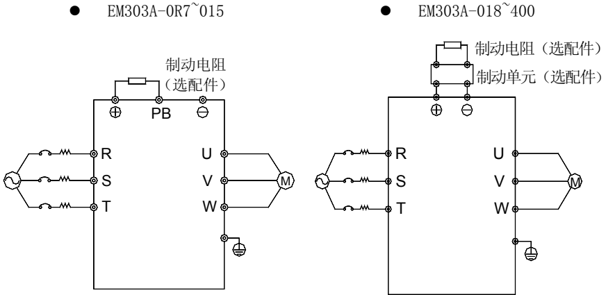
图 3-3 主回路标准接线
