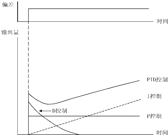
图 7-15 PID 控制的作用
