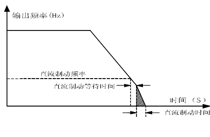
图 7-13 停车直流制动过程
