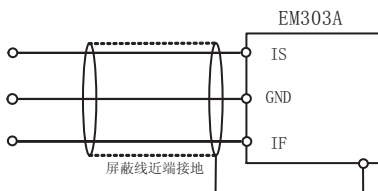
图 3-13 IS、IF 端子配线图
