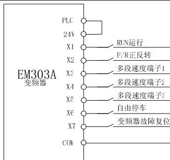
图 7-1 端子控制接线
