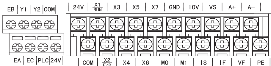
图 3-11 控制回路端子排列
