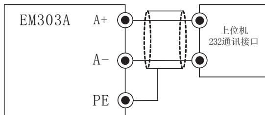
图 3-15 通讯端子配线
