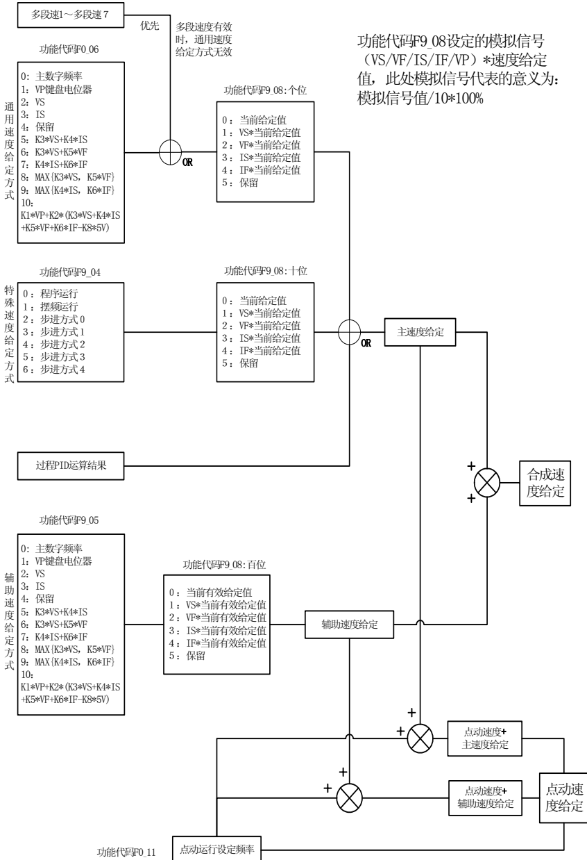
图 1-1 速度输入方式示意图
