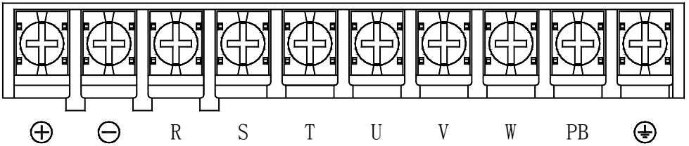
b. 主回路端子
