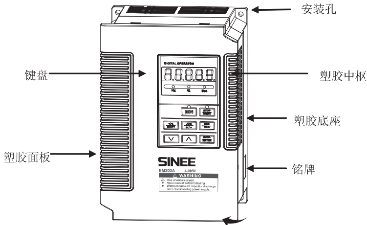
图 1-4 EM303A 系列变频器外型及部件
