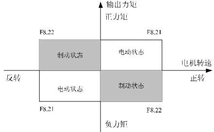
图 7-21 电动/制动力矩电流限定
