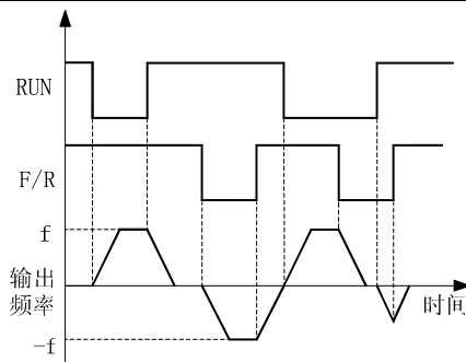
(d) F0.20=0, F0.05=1 正/反转运行逻辑
