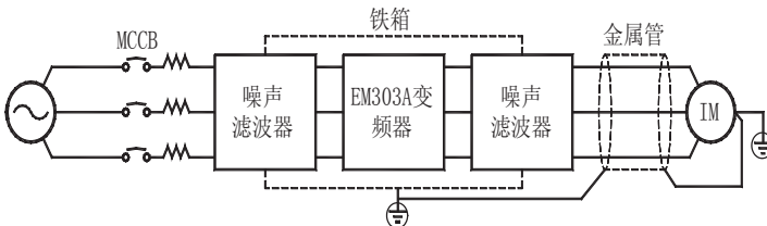
图 3-9 射频干扰对策
