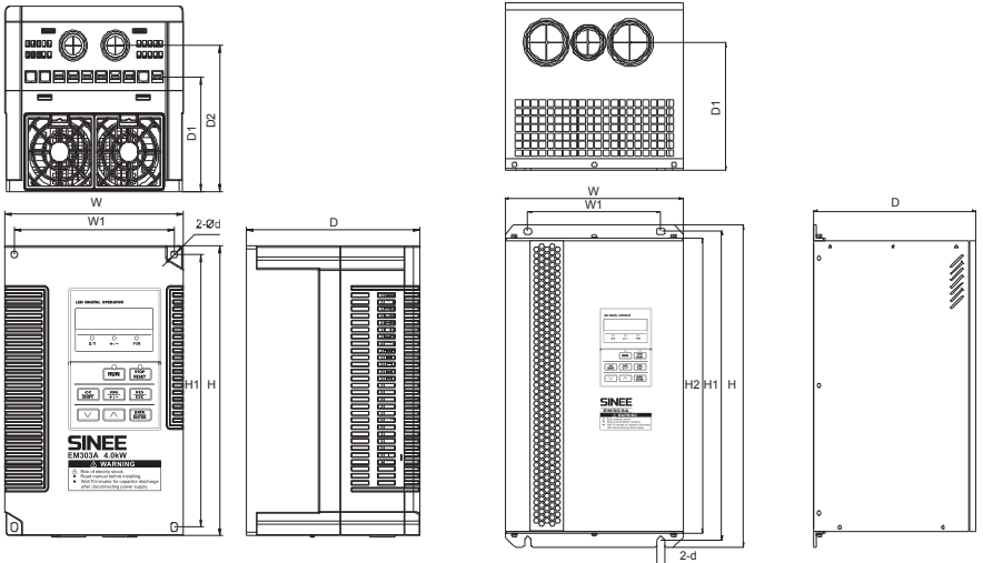
图 2-1 EM303A 系列开环矢量控制变频器和键盘外形尺寸图
