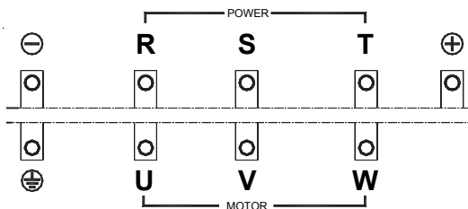
(c) 90kW 及以上规格主回路端子
