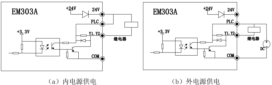
图 7-8 可编程端子供电方式
