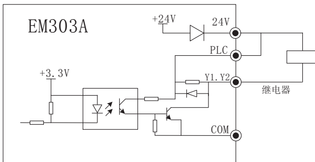
图 3-13 (a) 多功能输出端子用内部电源接线方式
