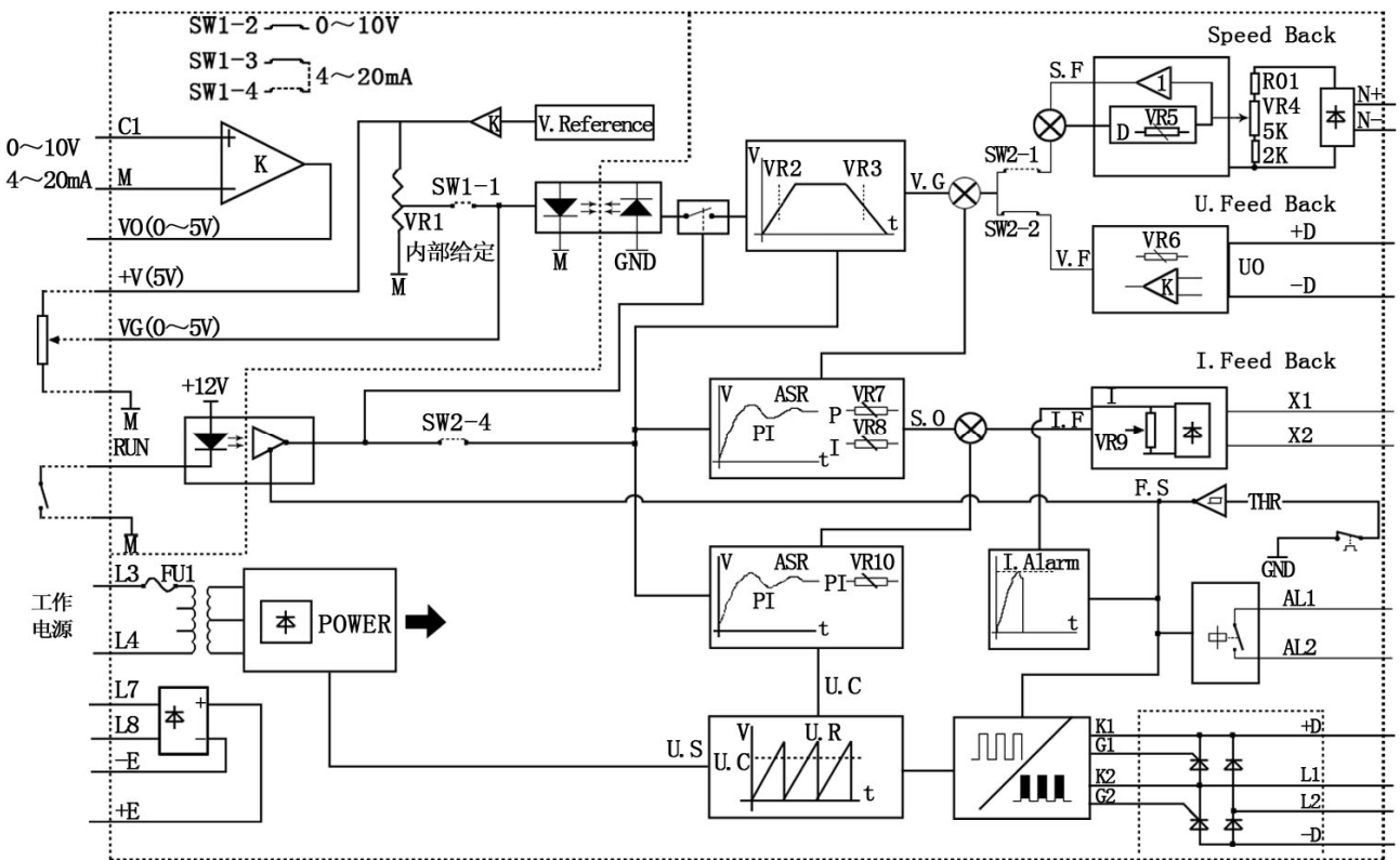
图 3-3 连接框图
