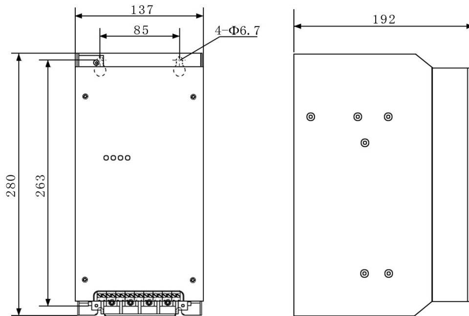
图 2-5 JK1-TS-□50、75、100
