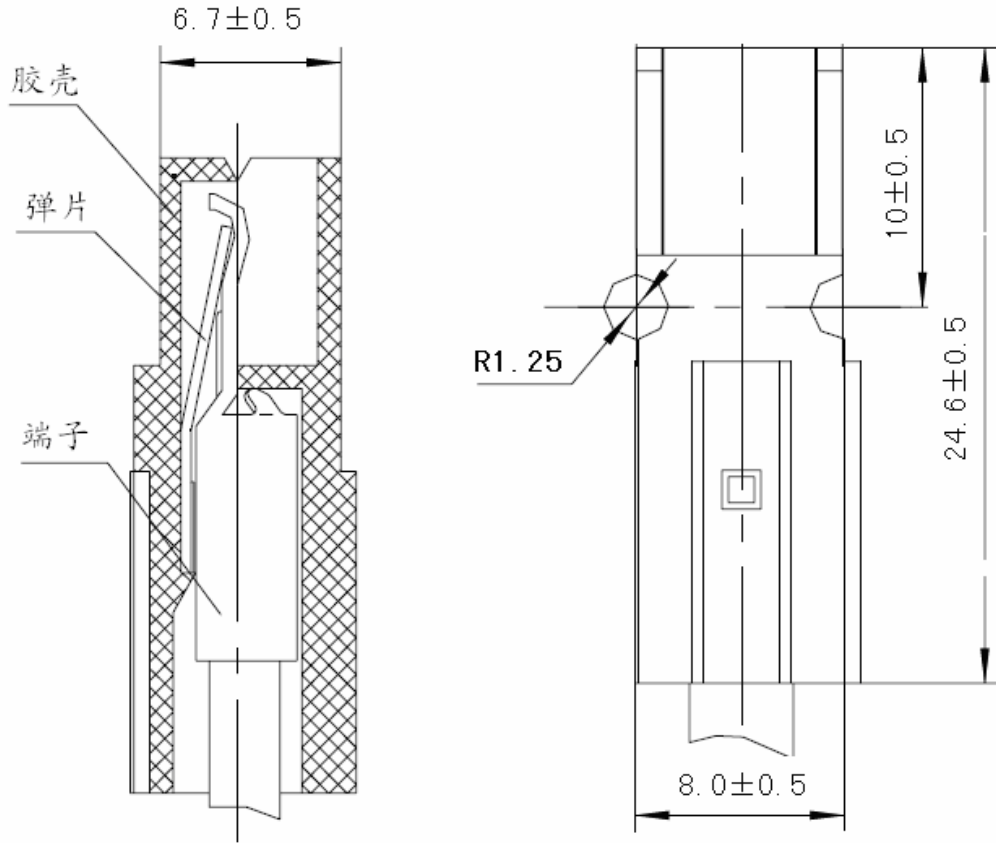
成品组装图+胶壳主要尺寸
