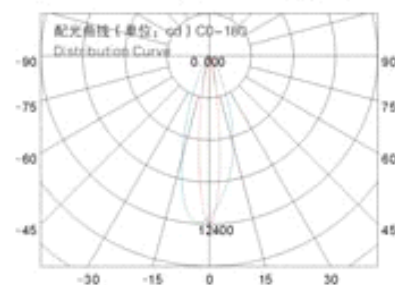
24x1W Cree Xlamp XP-E-Q5
