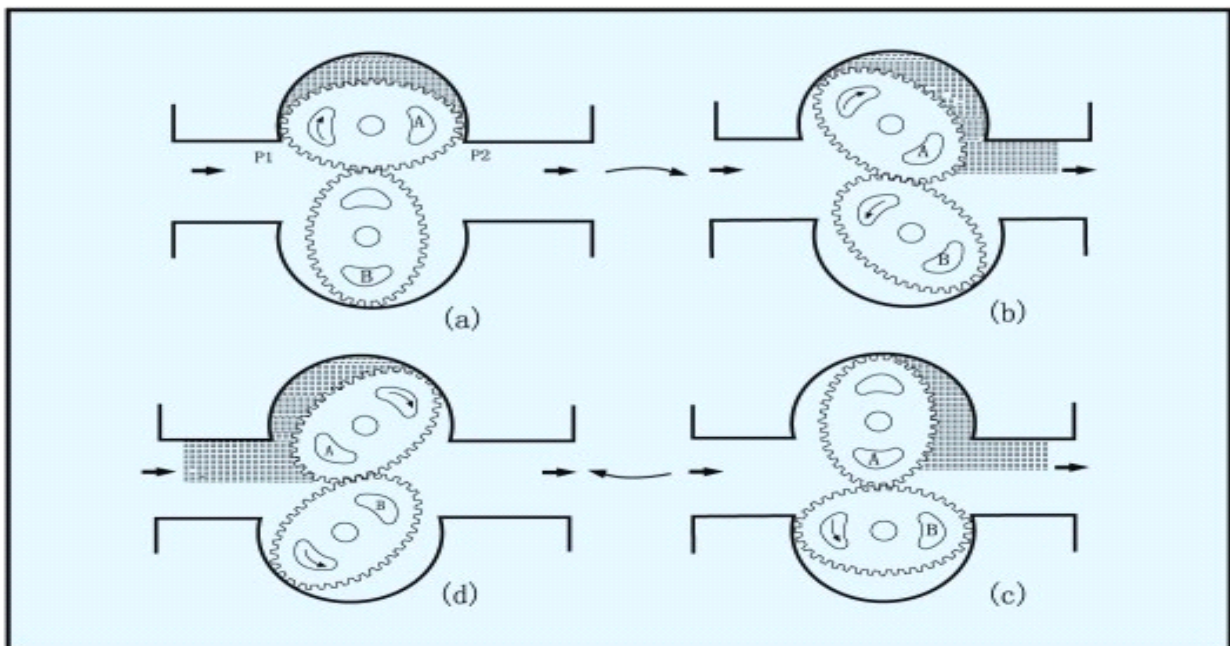
图 1 工作原理图
