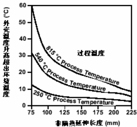
图 1 变送器外壳温度升高与用于测试安装的非隔热延伸长度的关系
