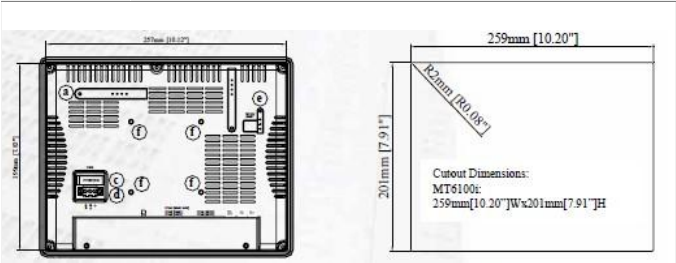
开孔尺寸
