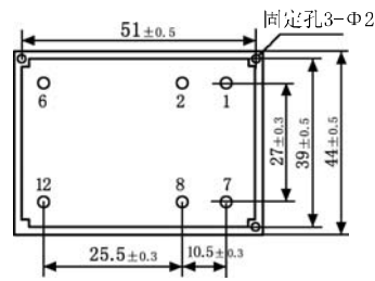
底视图 (单路输出)
