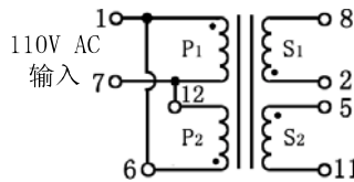
110V AC 输入接线图
