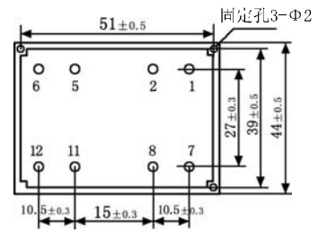
底视图 (双路输出)
