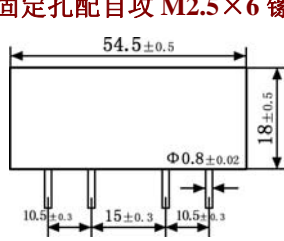
主视图
