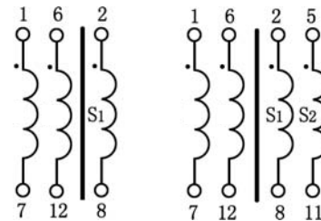
单路输出
