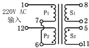
220V AC 输入接线图
