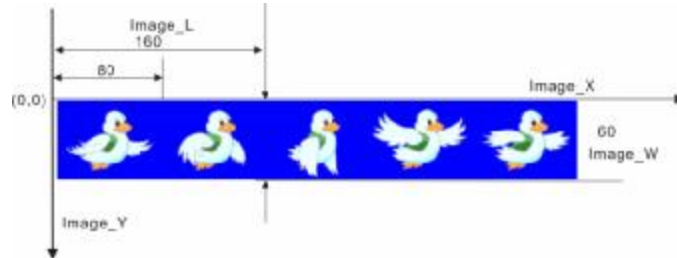
图 5.6 图片剪切参数说明
