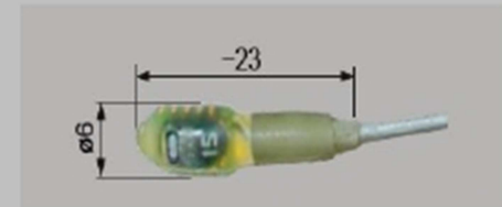
扩展湿度传感器
