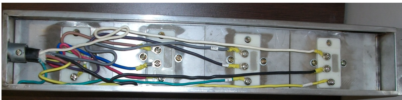
3、防窃电互感器底座接线图
