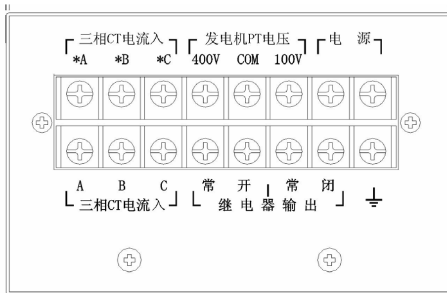
注：三相电流端同一侧为CT的同名端。 背板接线图
