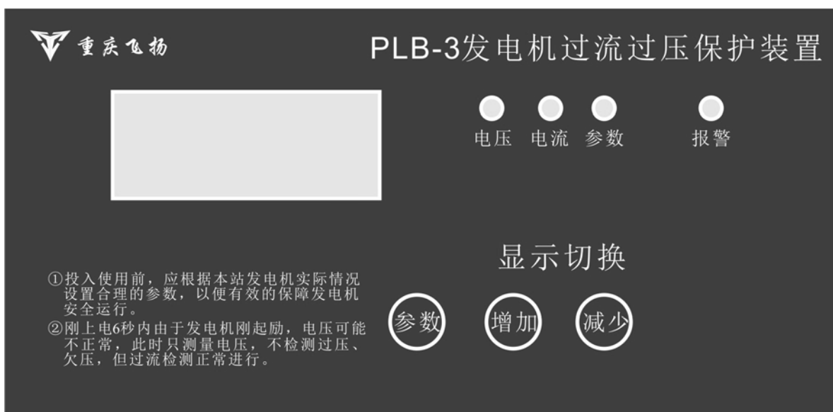
装置面板示意图
