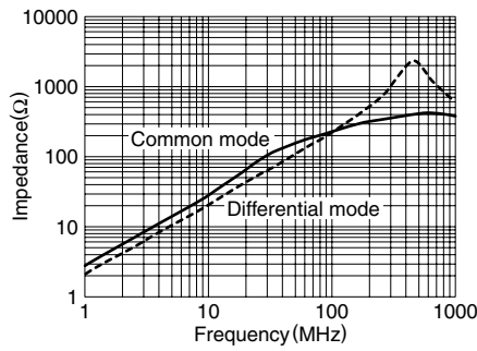
ACM1211-701-2PL
