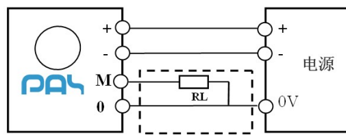
接线示意图
