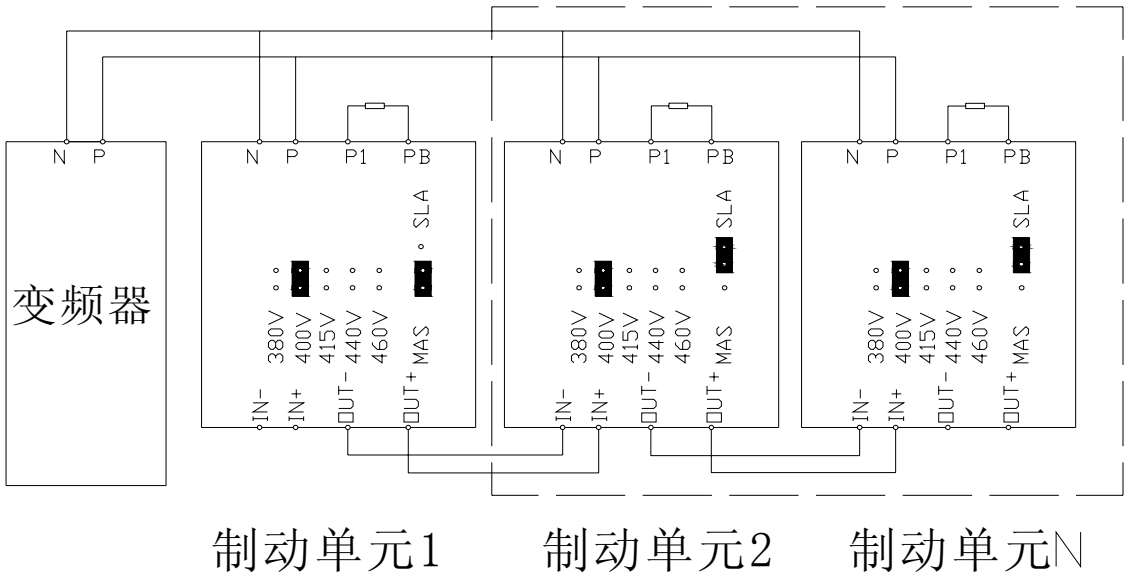
多台并联接线图
