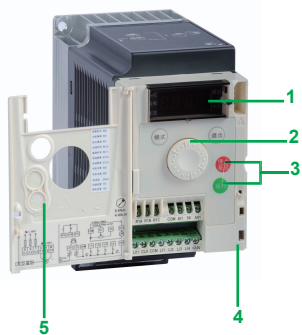
ATV303H037N4 带有门盖的前面板
