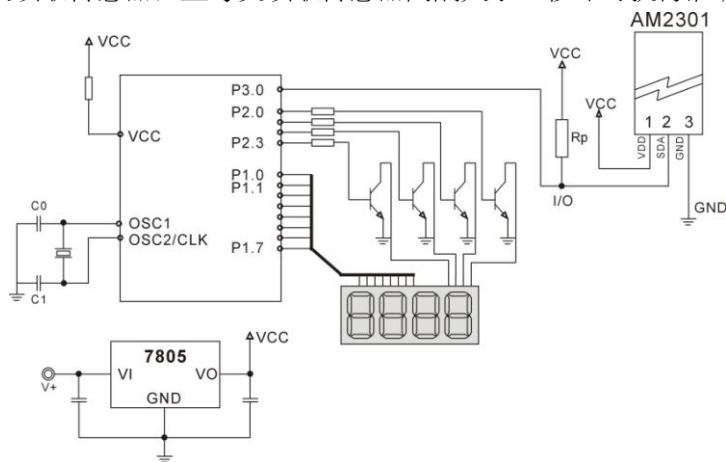
图 4： AM2301 单总线典型电路
