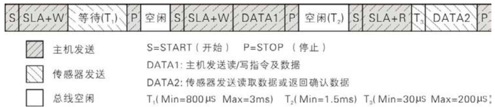
图 13: I 2 C 读写传感器完整示例图
