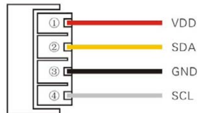
图 1：AM2311 接线图
