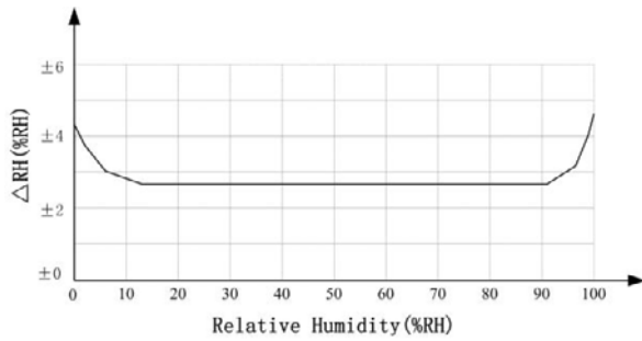
图 2: 25°C时 AM2311 的相对湿度最大误差
