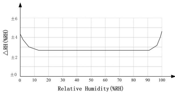
图 2: 25°C 时 AM2312 的相对湿度最大误差
