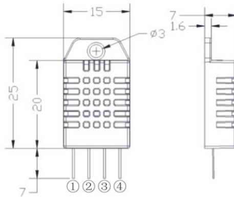
外形尺寸（单位：mm）
