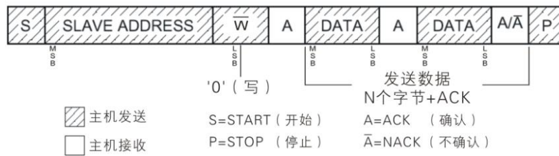
图 10: I 2 C 总线主机向从机发送数据基本格式
