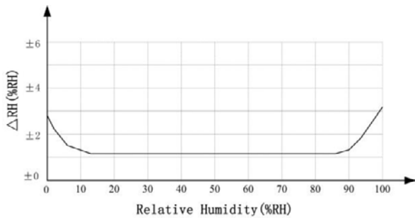
图 2: 25°C时 AM2315 的相对湿度最大误差
