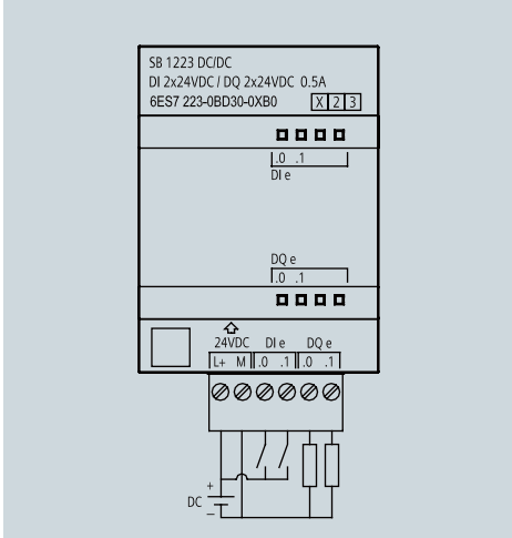
SB 1223 2 x 24 V DC 输入/2 x 24 V DC 输出接线图
