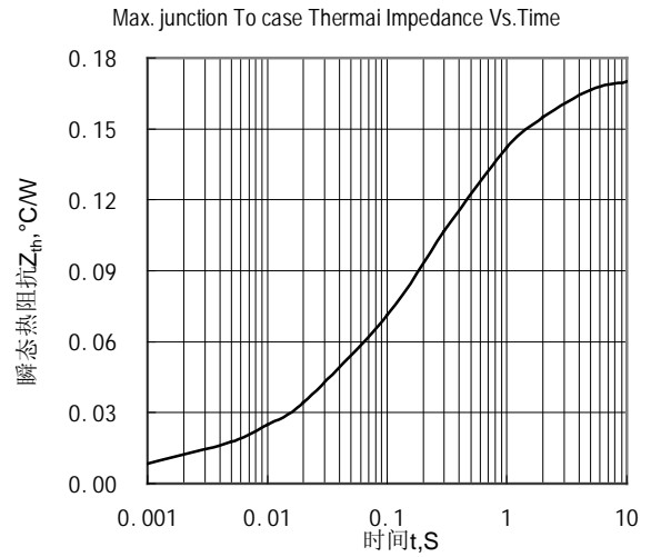
Fig.2 結至管殼瞬態熱阻抗曲線
