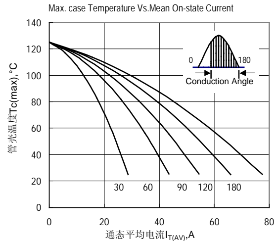
Fig.4 管殼溫度與通態平均電流關係曲線
