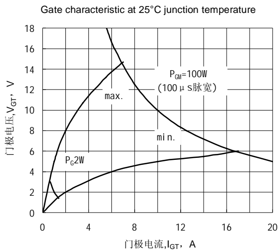
Fig.9 門極功率曲線
