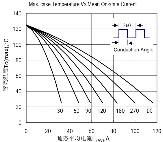
Fig.6 管殼溫度與通態平均電流關係曲線
