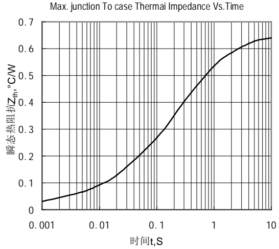
Fig.2 結至管殼瞬態熱阻曲線
