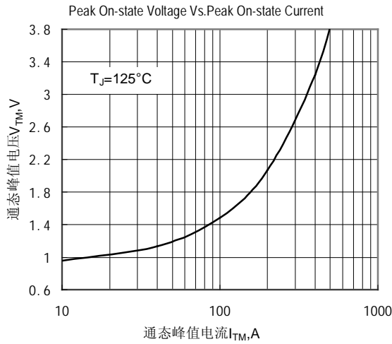
Fig.1 通態伏安特性曲線
