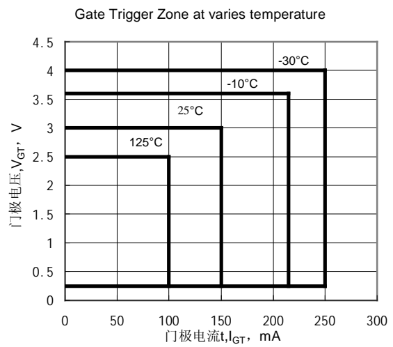
Fig.10 門極觸發特性曲線
