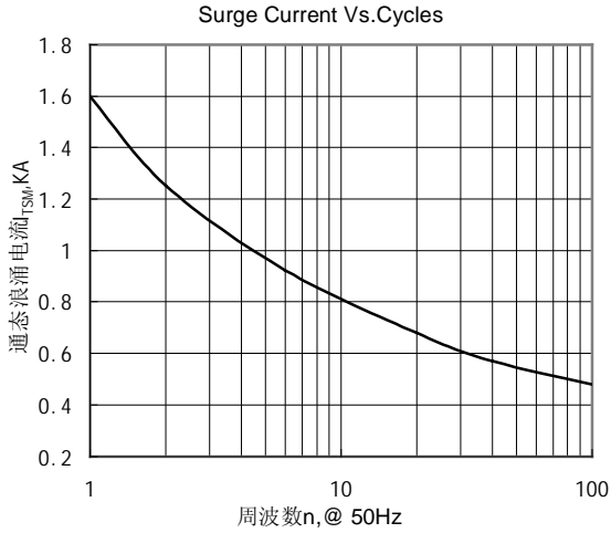
Fig.7 通態浪涌電流與周波數的關係曲線
