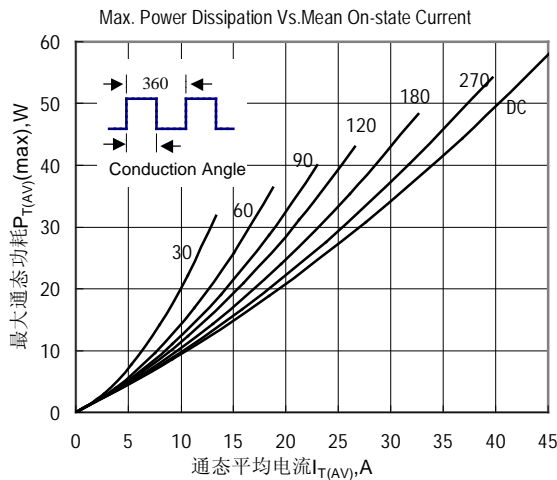
Fig.5 最大功耗與平均電流關係曲線
