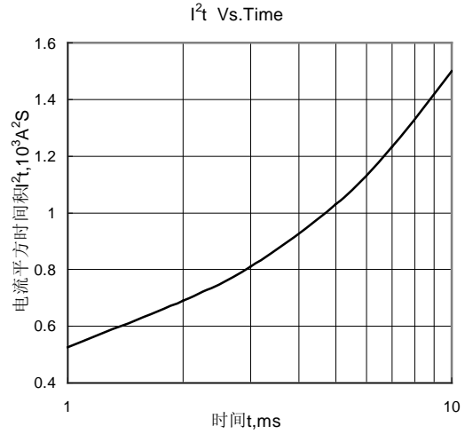
Fig.8 I^2t 特性曲線
