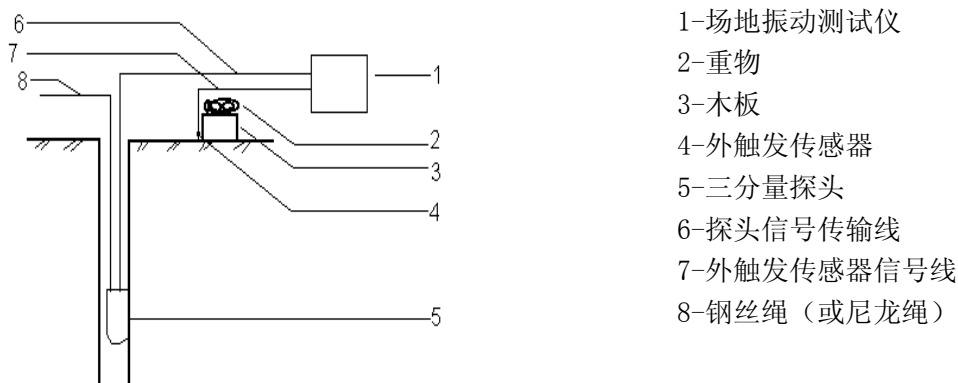
图 4 单孔波速测试示意图
