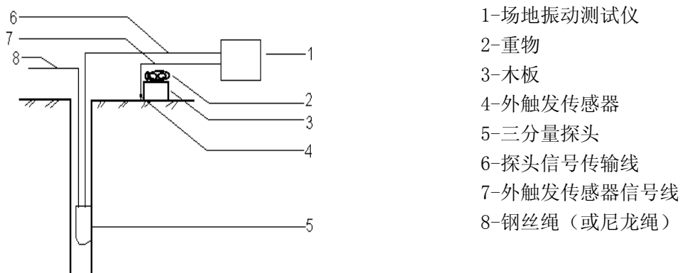
图 1 单孔波速测试示意图
