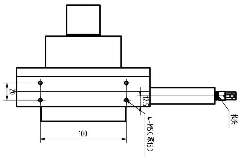
安装尺寸
