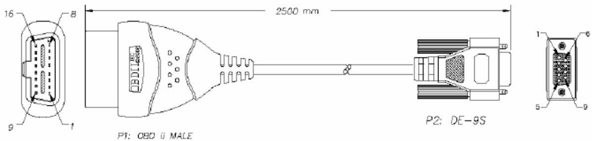
Kvaser OBD II Adapter Cable
