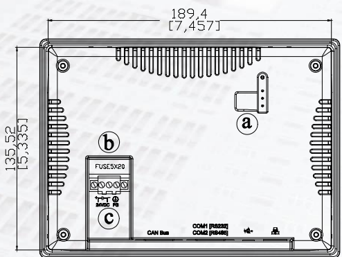
背视图
