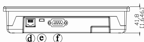
底视图
