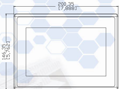
正视图
